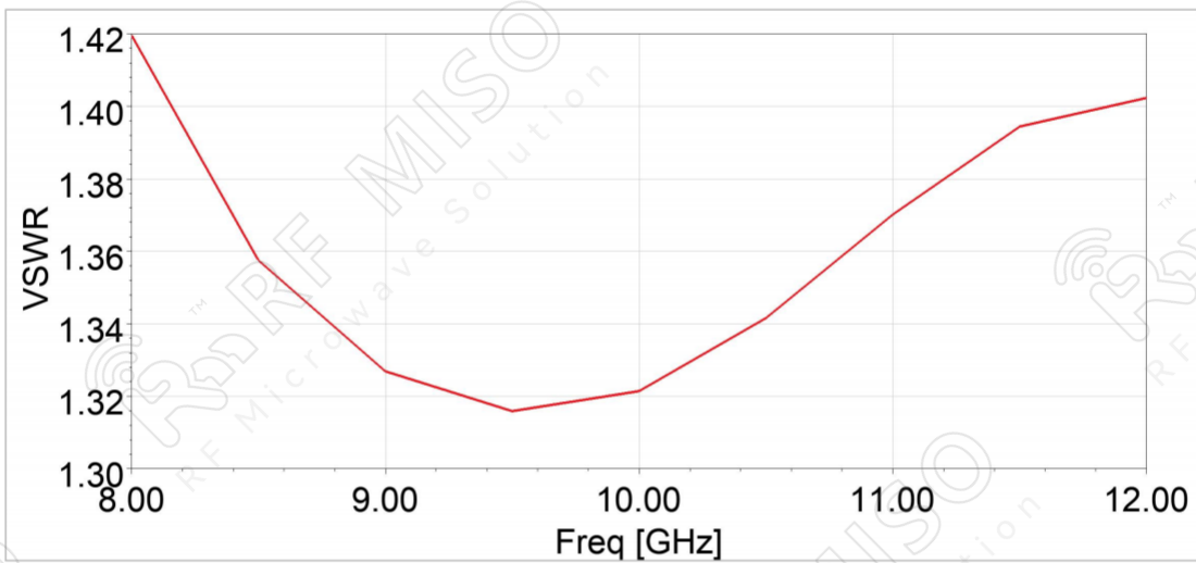
VSWR
