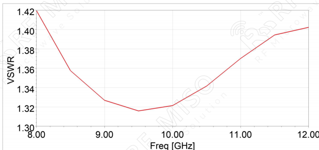
VSWR
