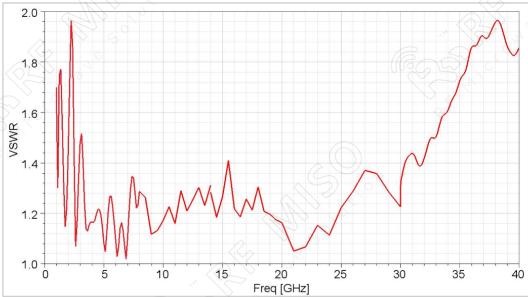
VSWR
