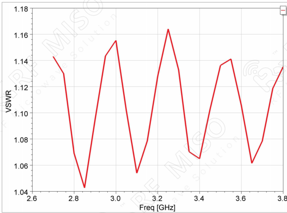
VSWR
