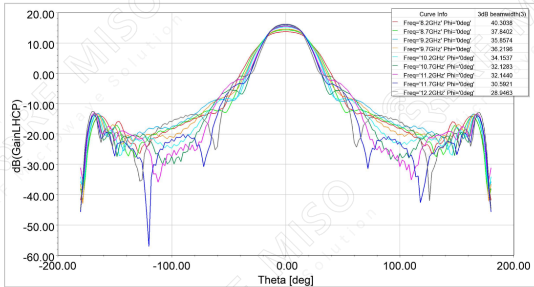
3dB Beamwidth
