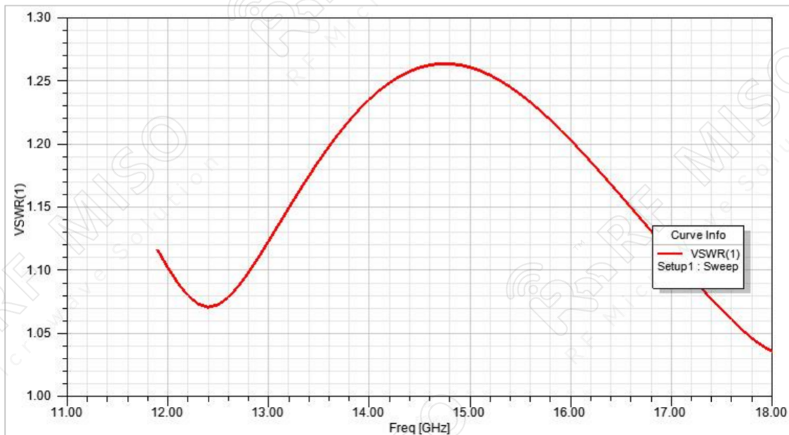
VSWR
