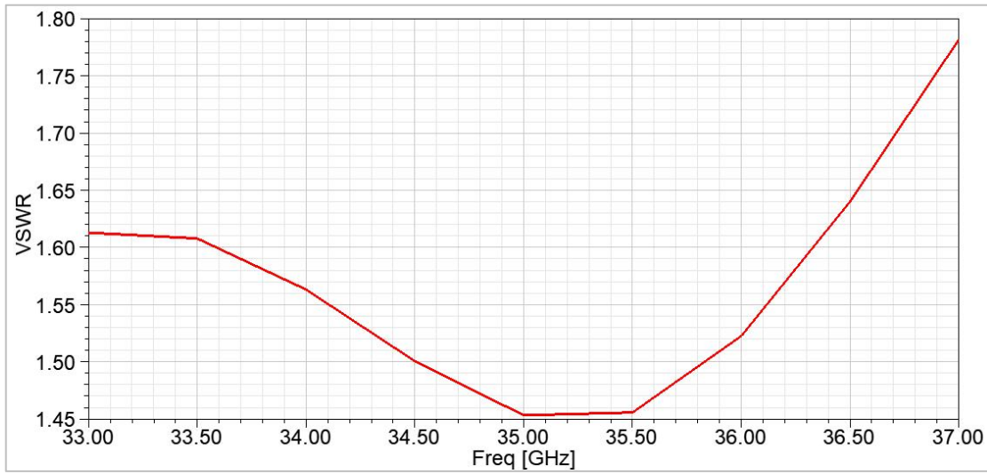
VSWR
