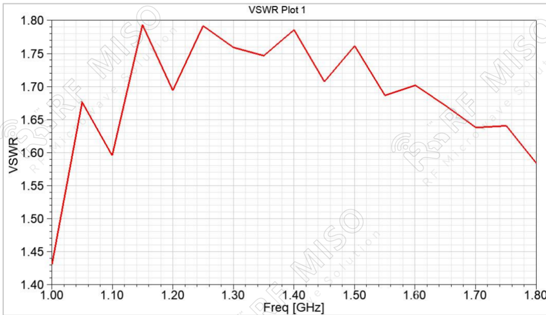
VSWR
